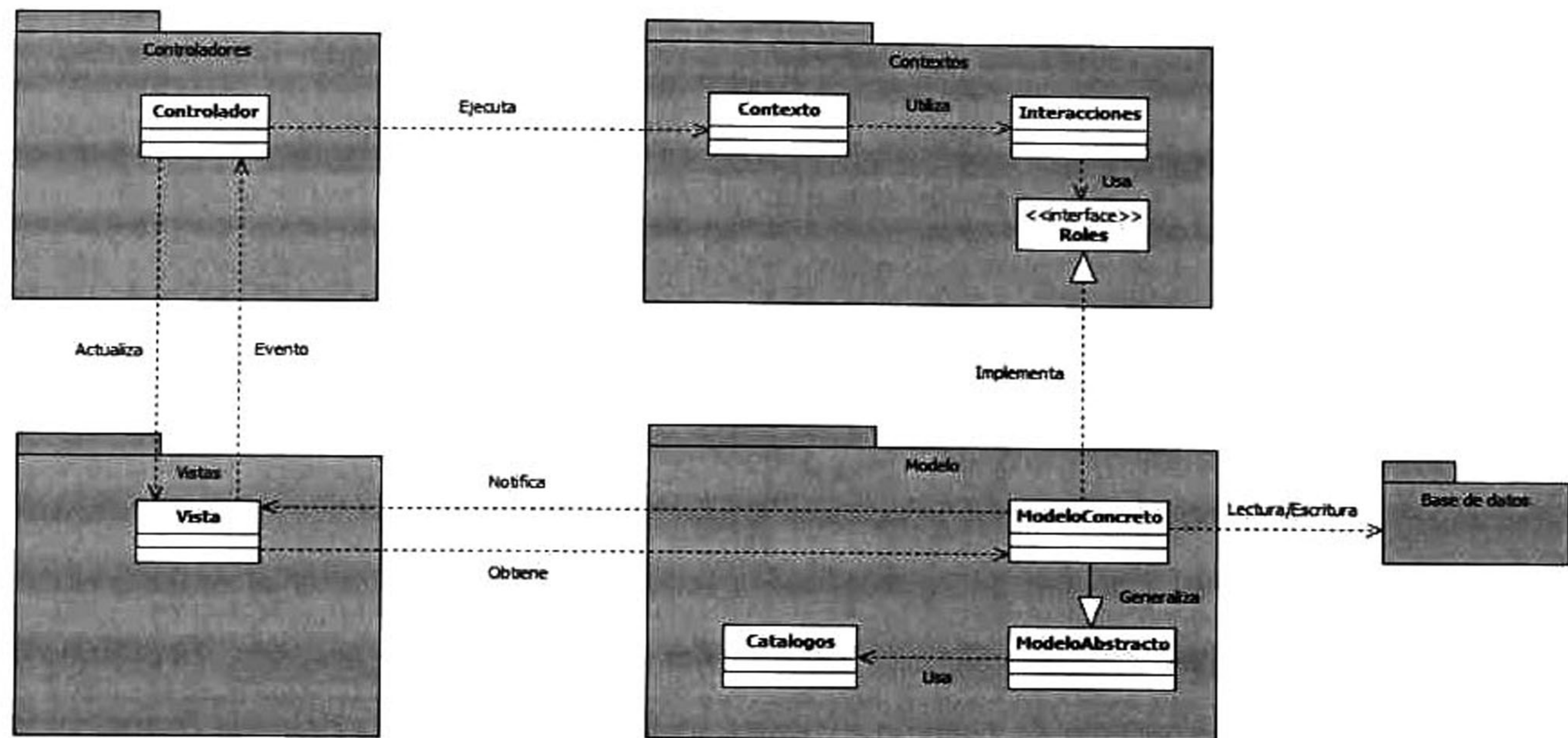
Figura 3.3: Vista modular del patrón arquitectónico DCI.
