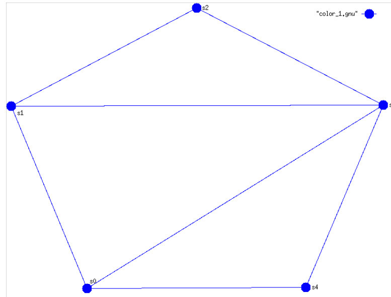
Figura 5.4: Clase cromática de color 1 para conjunto de puntos de tamaño n = 5 en posición convexa.
