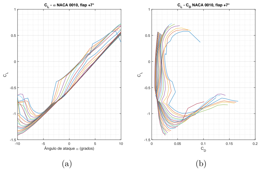
Figura 3.19: Gráficas C_L - \alpha (a) y C_L - C_D (b) para el perfil NACA 0010 con flap a +7^\circ .
