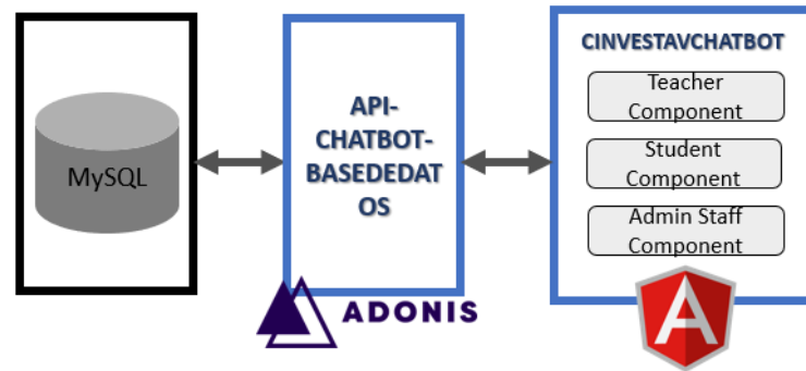
Figura 3.7: Proyecto API-CHATBOT-BASEDEDATOS.
