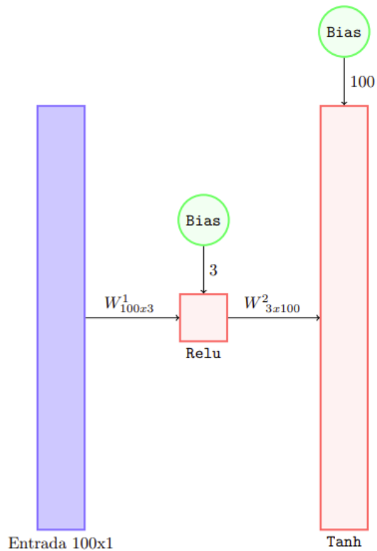
Figura 5.3: Esquema de un autoencoder elemental.
