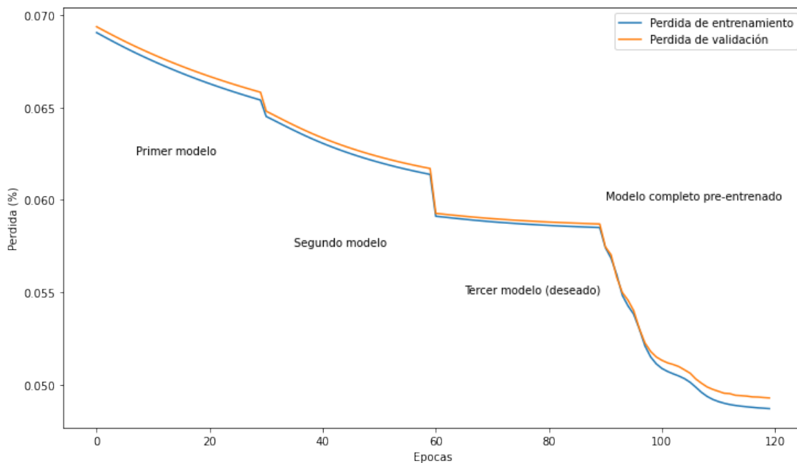
Figura 5.13: Curva de entrenamiento de las 4 etapas.
