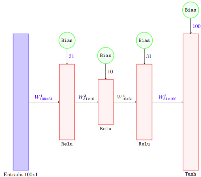
Figura 5.11: Segundo modelo. Parámetros color azul: Variables congeladas. Parámetros color negro: Variables entrenables.
