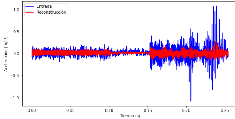
Figura 5.18: Gráficas de señal original ( gráfica azul ) y reconstrucción ( gráfica roja ).
