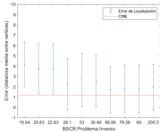
(f) Error en la localización de la fuente de actividad neuronal con BSCR = 80 y SNR = 10%.
