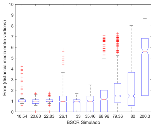
(c) Error en la localización de la fuente de actividad neuronal de diferentes BSCR: Dipolo 2 (visual), SNR 1 %.
