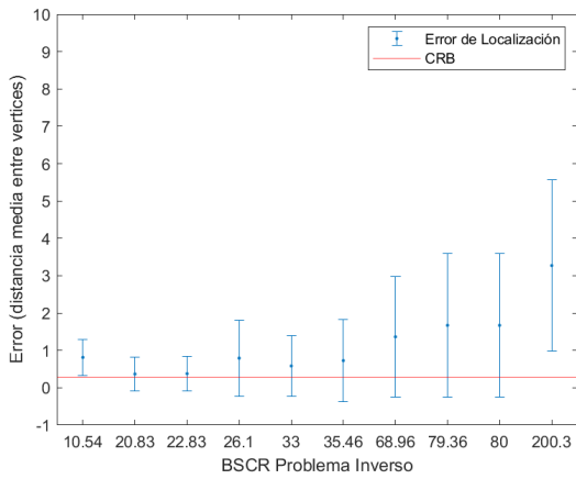
(c) Error en la localización de la fuente de actividad neuronal con BSCR = 20 SNR = 5%.
