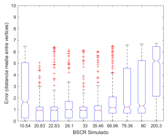
(f) Error en la localización de la fuente de actividad neuronal de diferentes BSCR: Dipolo 3 (auditiva), SNR 10 %.
