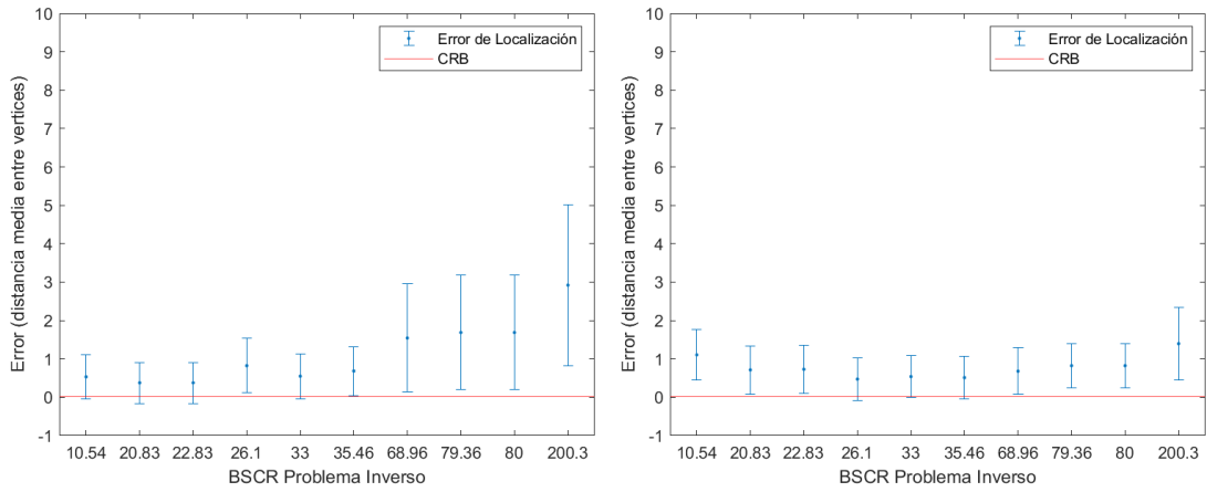
(a) Error en la localización de la fuente de actividad neuronal con BSCR 10. (b) Error en la localización de la fuente de actividad neuronal con BSCR 20.
